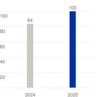
Tendenza NPS
